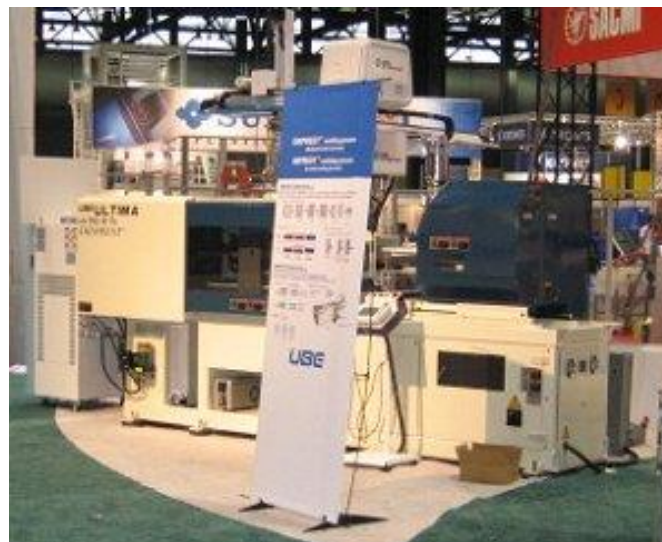
UN110us 全電動式ダイプレスト射出成形機
